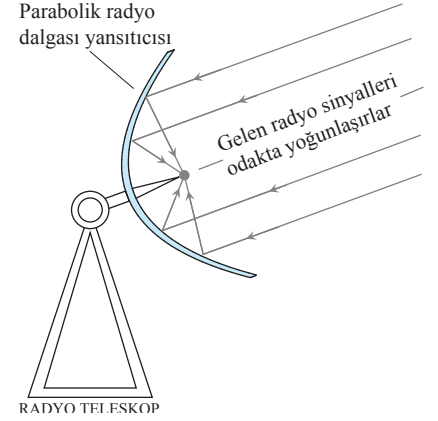
ŞEKİL 10.14 Parabolik yansıtıcılar, odaklarındaki bir kaynaktan gelen ışınları, parabol eksene paralel bir ışık demetine dönüştürebilir; veya, eksene paralel gelen ışınları toplayıp odakta yoğunlaştırırlar.
