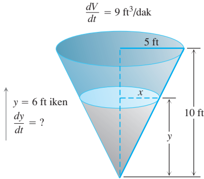
ŞEKİL 3.45 Konik tankın geometrisi ve suyun tankı doldurma oranı, su seviyesinin ne hızla yükseldiğini belirler (Örnek 4).
