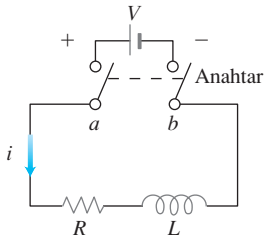
ŞEKİL 9.5 Örnek 5'teki RL devresi.
