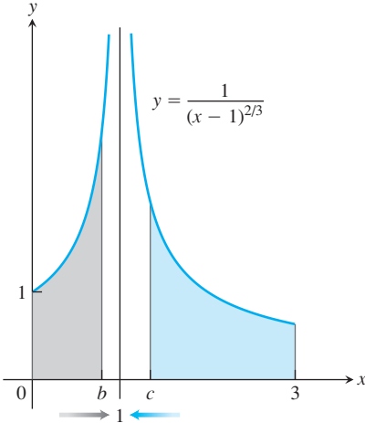
ŞEKİL 8.23 Örnek 5
