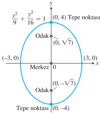
ŞEKİL 10.9 Asal eksen dikey olan bir elips (Örnek 3).
