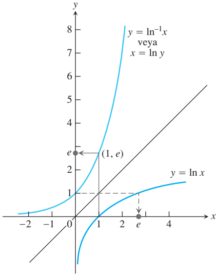
ŞEKİL 7.11 y = \ln x ve y = \ln^{-1} x = \exp x 'in grafikleri. e sayısını \ln^{-1} 1 = \exp(1) dir.
