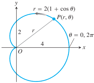
ŞEKİL 10.50 Örnek 1'deki kardoid.
