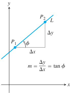
ŞEKİL 1.11 Dikey olmayan bir doğrunun eğimi, eğim açısının tanjantıdır.
