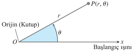
ŞEKİL 10.35 Düzlem için kutupsal koordinatları tanımlamak üzere, kutup denilen bir orijin ve bir başlangıç ışınıyla işe başlarız.
