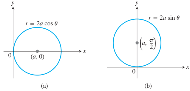
ŞEKİL 10.59 Orijinden geçen, a yarıçaplı ve merkezi (a) pozitif x -ekseninde (b) pozitif y -ekseninde olan bir çemberin kutupsal denklemleri.
