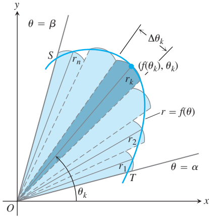
ŞEKİL 10.48 OTS bölgesinin alanının bir formülünü bulmak için, bölgeye pervane şekilli dairesel kesitlerle yaklaşımda bulunuruz.
