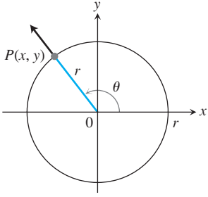
ŞEKİL 1.68 Genel bir \theta açısının trigonometrik fonksiyonları x , y ve r cinsinden tanımları.
