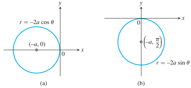
ŞEKİL 10.60 Orijinden geçen, a yarıçaplı ve merkezi (a) negatif x -ekseninde (b) negatif y -ekseninde olan bir çemberin kutupsal denklemleri.
