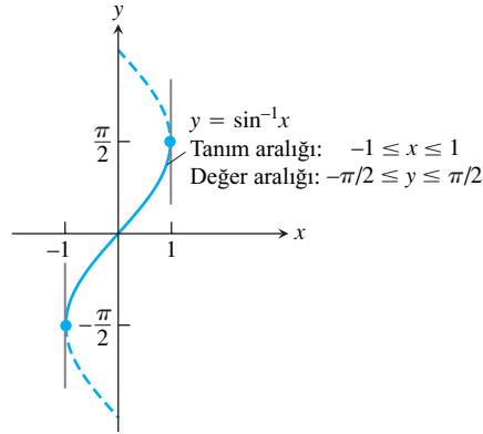
ŞEKİL 7.29 y = \sin^{-1} x 'in grafiği.
