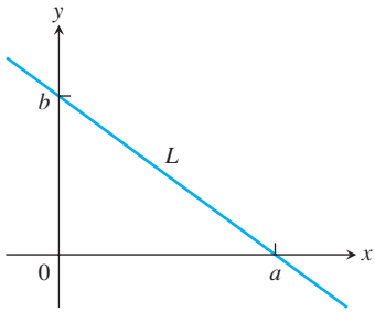
ŞEKİL 1.14 L doğrusunun x-kesimi a ve y-kesimi b dir.
