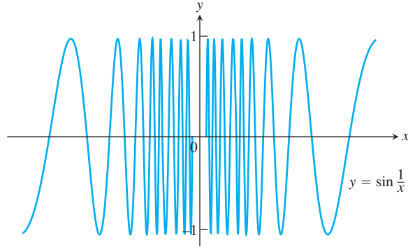
ŞEKİL 2.28 y = \sin(1/x) fonksiyonunun x sıfıra yaklaşıırken sağdan veya soldan limiti yoktur (Örnek 4).
