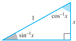
ŞEKİL 7.21 \sin^{-1} x ve \cos^{-1} x are bütünleyen açılardır (dolayısıyla toplamaları \pi/2 'dir).
