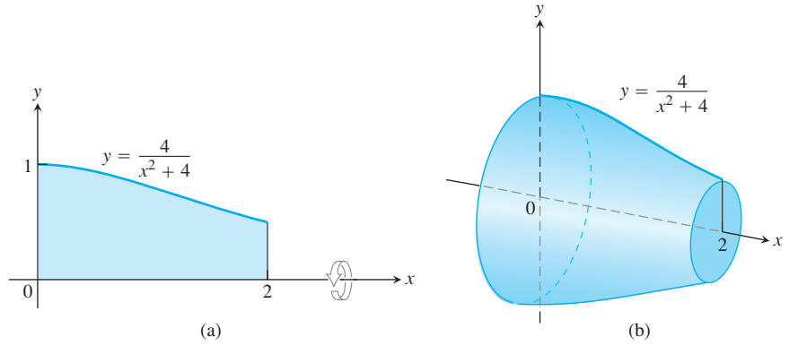
ŞEKİL 8.7 Örnek 4'teki bölge (a) ve dönel cisim (b).
