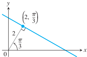
ŞEKİL 10.57 Bu doğrunun standart kutupsal denklemini x + \sqrt{3}y = 4 Kartezyen denklemine dönüştür (Örnek 1).
