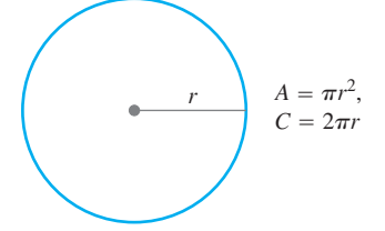
Çember
