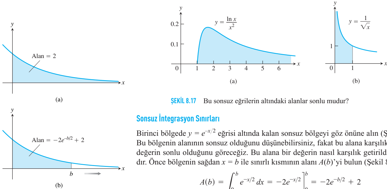
ŞEKİL 8.18 (a) Birinci bölgede y = e^{-x/2} eğrisinin altındaki alan (b) birinci tipte bir genelleştirilmiş integraldir.
