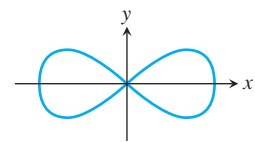
42. Lemniskat
