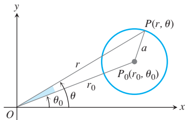
ŞEKİL 10.58 Bu çemberin kutupsal denklemini, Kosinüs Kuralını OP_0P üçgenine uygulayarak bulabiliriz.
