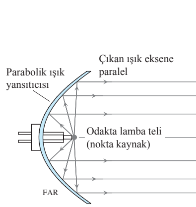
ŞEKİL 10.14 Parabolik yansıtıcılar, odaklarındaki bir kaynaktan gelen ışınları, parabol eksene paralel bir ışık demetine dönüştürebilir; veya, eksene paralel gelen ışınları toplayıp odakta yoğunlaştırırlar.
