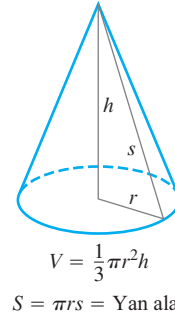
Dik Dairesel Koni
