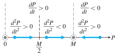
ŞEKİL 9.21 Lojistik büyüme için tamamlanmış faz doğrusu (Denklemler 6 ve 7).
