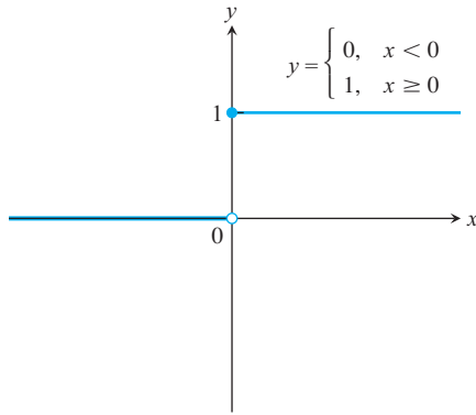
(a) Birim basamak fonksiyonu U(x)
