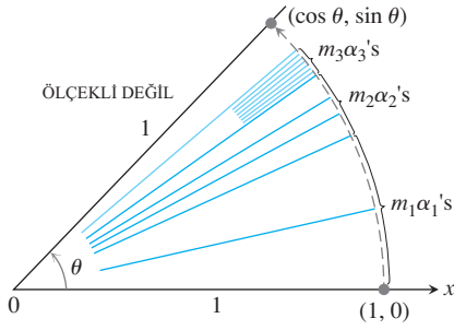
ŞEKİL 10.27 0 ile 2\pi arasındaki bir \theta açısının sinüs ve kosinüsünü hesaplamak için, hesap makinesi (1, 0) noktasını birim çemberde uygun bir konuma yerleştirir ve ortaya çıkan koordinatları gösterir.
