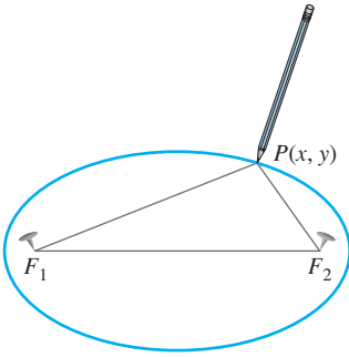
ŞEKİL 10.5 Bir elips çizmenin bir yolu, iki raptiye ve kaleme rehberlik eden bir ip kullanılır.
