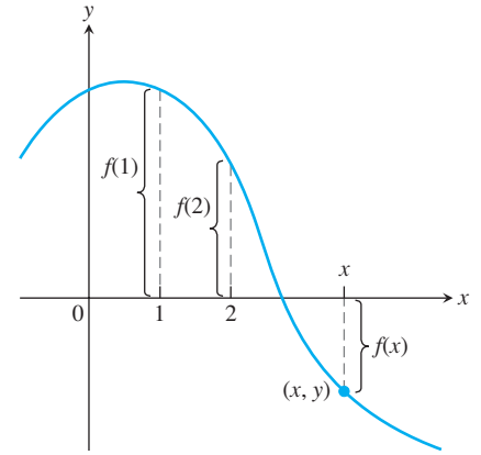
ŞEKİL 1.25 (x, y) noktası f 'in grafiği üzerinde ise y = f(x) değeri x noktasında grafiğin yüksekliğidir (veya f(x) negatif ise x noktasının altındaki yükseklik).
