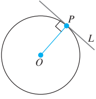
ŞEKİL 2.63 L doğrusu, P 'den OP yarıçapına dik olarak geçerse çembere teğettir.
