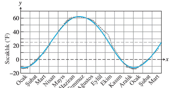
ŞEKİL 3.33 Fairbanks, Alaska'da hava sıcaklıkları normal ortalaması, veri noktaları olarak çizilmiş ve sinüs yaklaşım fonksiyonu (Alıştırma 96).
