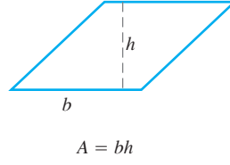
Paralelkenar
