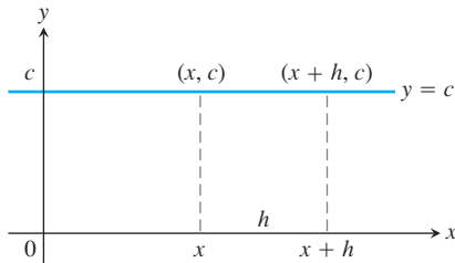
ŞEKİL 3.8 (d/dx)(c) = 0 kuralı sabit fonksiyonların değerlerinin asla değişmediğini ve yatay bir doğrunun eğiminin her noktada sıfır olduğunu söylemenin başka bir yoludur.
