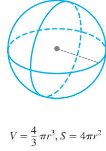
Küre
