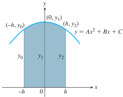
ŞEKİL 8.15 -h 'den h 'ye integre etmekle renkli alanı
