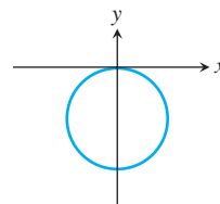
43. Çember
