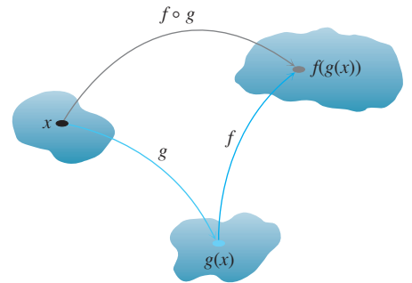
ŞEKİL 1.53 f \circ g için ok diyagramı.
