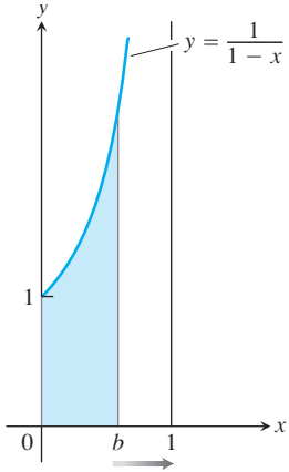
ŞEKİL 8.22 Limit yoktur:
