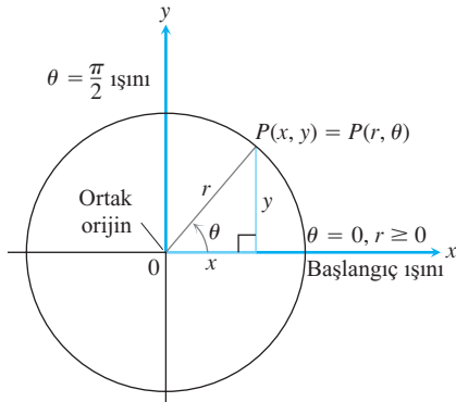
ŞEKİL 10.41 Kutupsal ve Kartezyen koordinatları birleştirmenin genel yolu.
