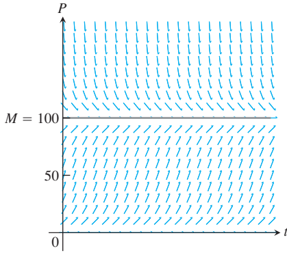
ŞEKİL 9.25 Lojistik diferansiyel denklem için bir eğim alanı dP/dt = 0.001(100 - P)P (Örnek 2).
