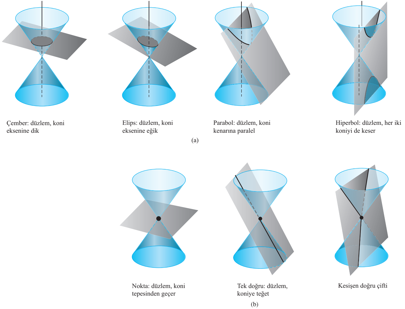
ŞEKİL 10.1 Standart konik kesitler (a) Bir düzlemin bir çift koniyi kestiği eğriler. Hiperbol, kollar denen iki bölümden oluşur. Nokta ve doğrular, düzlemin koni tepesinden geçirilmesi ile elde edilirler (b) dejenere konik kesitler.
