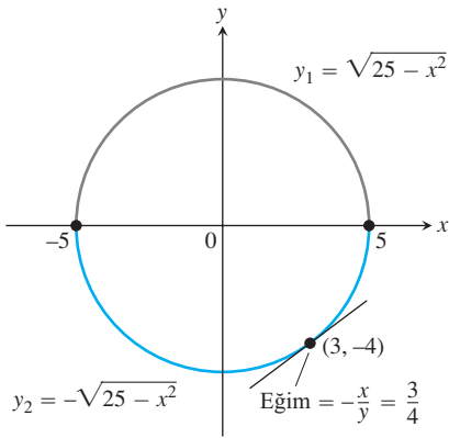
ŞEKİL 3.36 Çember iki fonksiyonun grafiklerini birleştirir. y_2 grafiği alt yarı çemberdir ve (3, -4) noktasından geçer.
