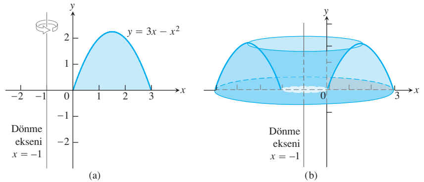
ŞEKİL 6.17 (a) Örnek 1'deki bölgenin grafiği, döndürülmeden önce. (a)'daki bölgenin x = -1 dönme eksen etrafında döndürülmesi ile oluşan cisim.
