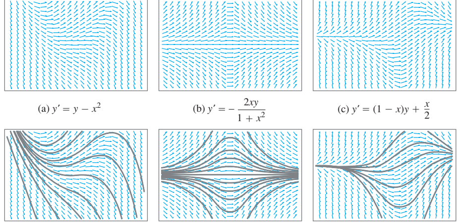
ŞEKİL 9.3 Eğim alanları (üst satır) ve seçilmiş çözüm eğrileri (alt satır). Bilgisayar gösterimlerinde eğim parçaları, burada olduğu gibi, bazen oklarla resmedilirler. Ancak bu, eğimlerin yönleri olduğu şeklinde algılanmamalıdır, çükü yoktur.
