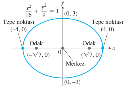
ŞEKİL 10.8 Asal eksen yatay olan bir elips (Örnek 2).
