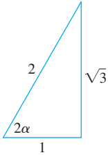
ŞEKİL 10.25 2\alpha = \cot^{-1}(1/\sqrt{3}) 'ü \pi/3 olarak tanımlar (Örnek 2).
