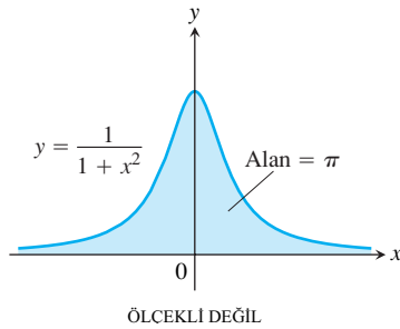
ŞEKİL 8.20 Bu eğrinin altındaki alan sonludur (Örnek 2).
