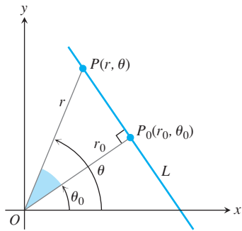
ŞEKİL 10.56 OP_0P dik üçgeninden r_0 = r \cos(\theta - \theta_0) bağıntısını okuyarak L doğrusunun bir kutupsal denklemini elde edebiliriz.
