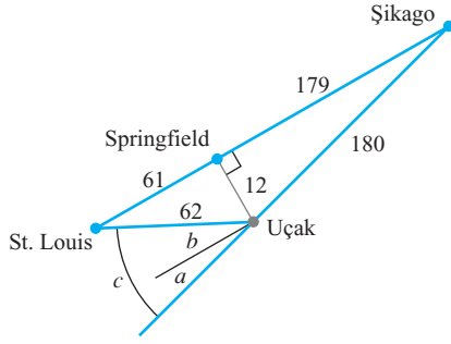
ŞEKİL 7.28 Uzaklıklar mil olarak yuvarlanmış şekilde kayma düzeltmesi (Örnek 7) diyagramı (çizim ölçekli değil).
